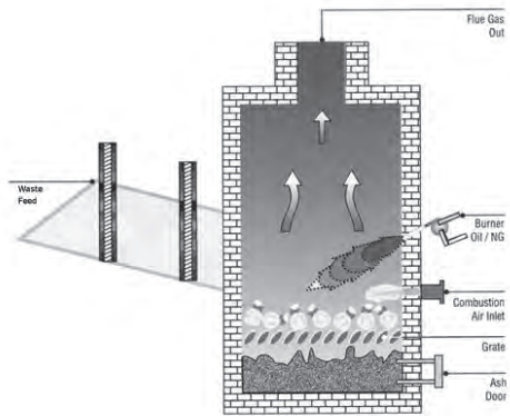
Ilustración 46: Proceso de incineración. Fuente: Pacific Consultants & Engineers.
